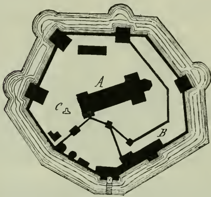
126. NAGYVÁRAD VÁRÁNAK TERVRAJZA.
